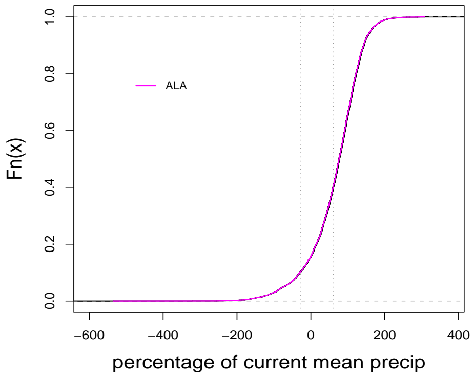
Delta P, DJF
