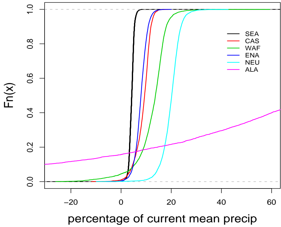
Delta P, DJF
