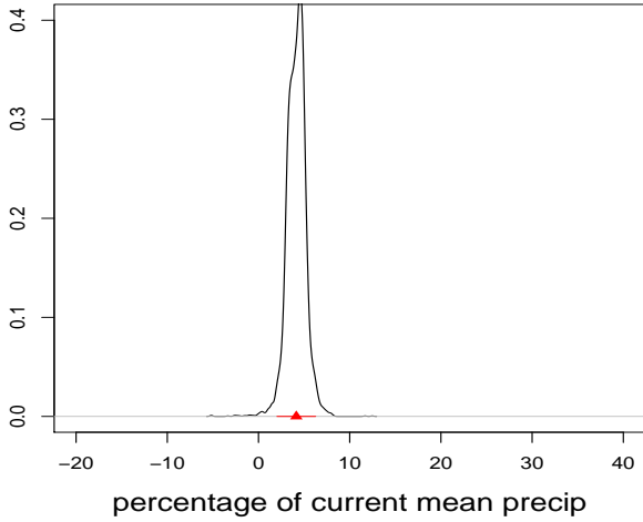
SEA: Delta P, DJF
