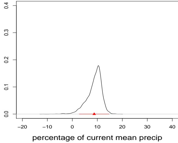
CAS: Delta P, DJF
