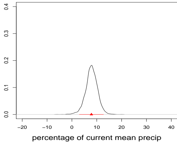
ENA: Delta P, DJF
