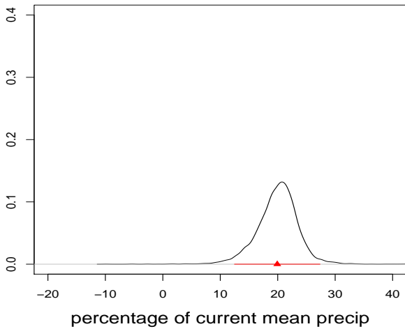
NEU: Delta P, DJF
