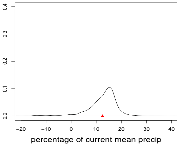
WAF: Delta P, DJF
