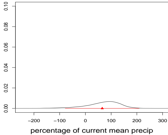
ALA: Delta P, DJF
