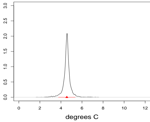
ENA: Delta T, DJF
