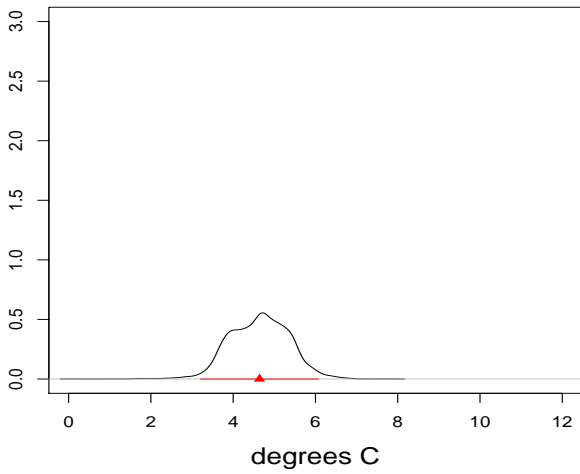
NEU: Delta T, DJF
