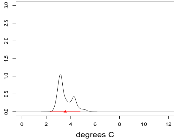
CAS: Delta T, DJF
